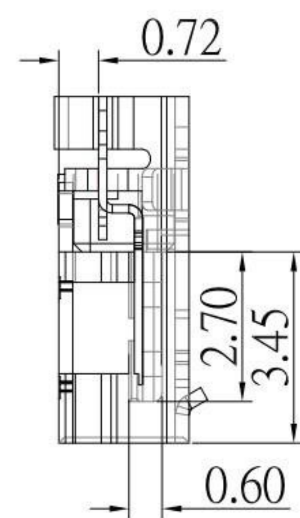
SEC A-A
