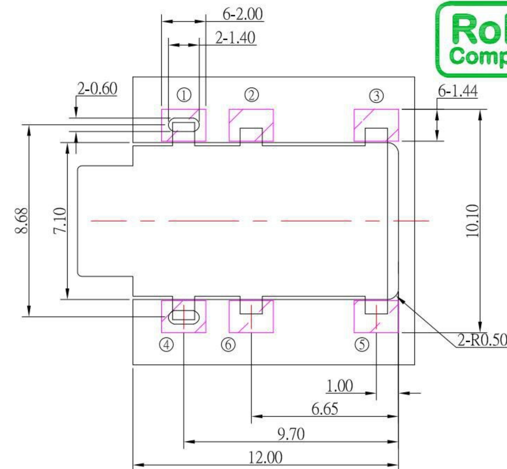
P.C.B LAYOUT
