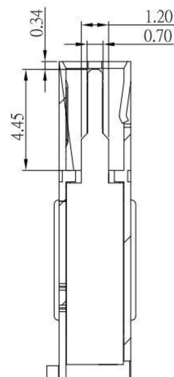
剖視圖
