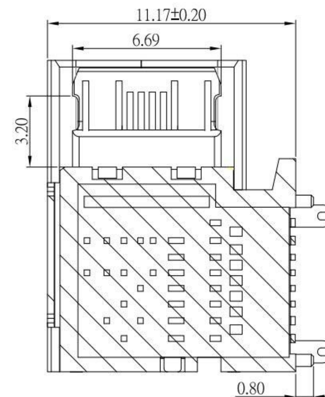
剖視圖
