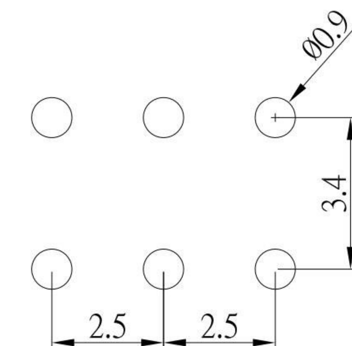
P.C.B LAND PATTERN
